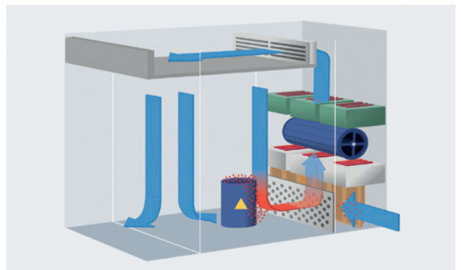
Grundprinzip zum Schutz des Bedieners und des Produkts
