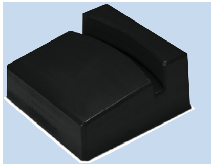
Fasskeil PE ermöglicht das Schrägstellen von 200-Liter-Stahl- und Kunststoff-Fässern optimale Entleerung des Fasses mittels Pumpe möglich B x T x H (mm): 217 x 214 x 97 Bestell-Nr. 12124
