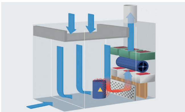
Grundprinzip zum Schutz des Bedieners
