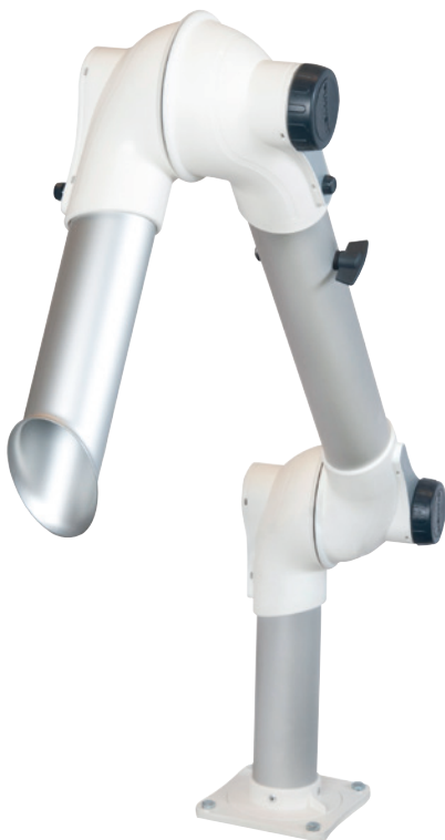
Quellenabsaugungen für das Labor zur direkten Tischmontage, Saugspitze optional Bestell-Nr. 10147
