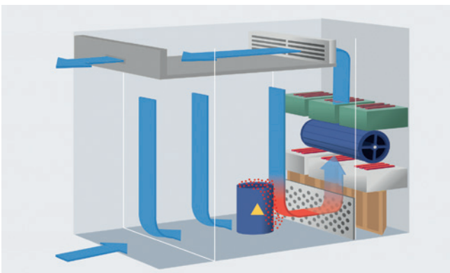
Grundprinzip zum Schutz des Bedieners
