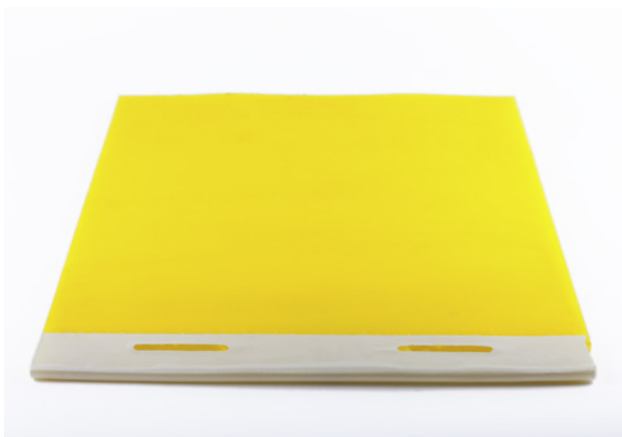
Abdichtmatte , B x T x H (mm): 800 x 800 x 8 Bestell-Nr. 13098
